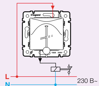
Переключатель без фиксации перекидной со шнуром Кат. № 7 744 19 - 7 743 19 - 7 701 19
